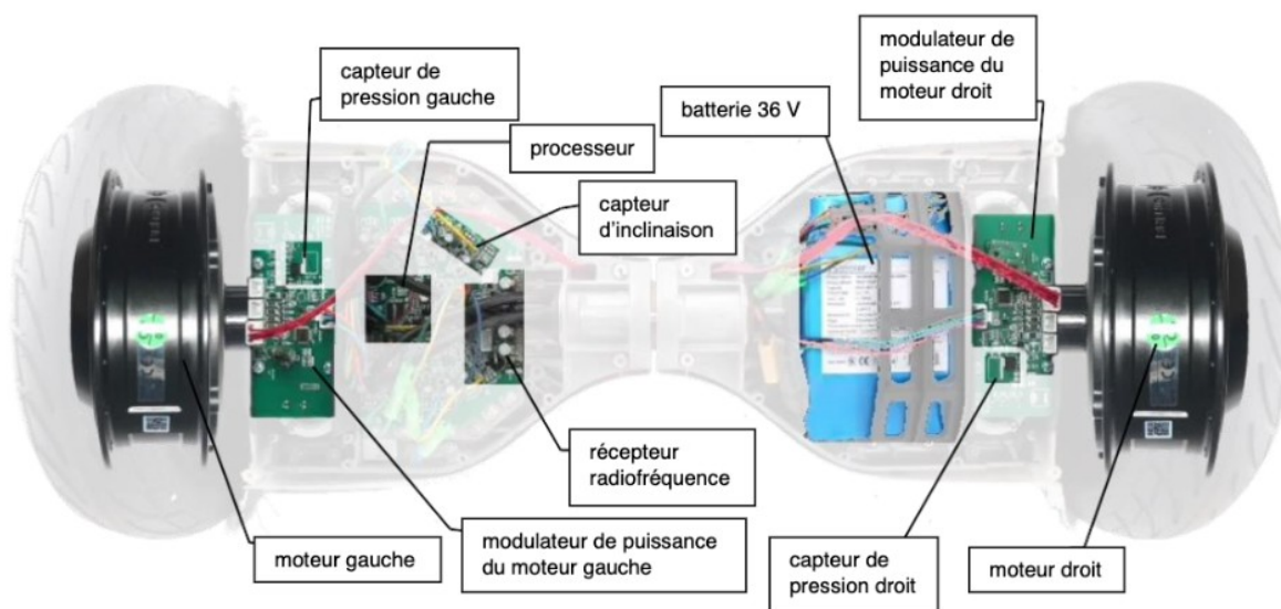
Figure 2 : vue interne de l'overboard Xenox
