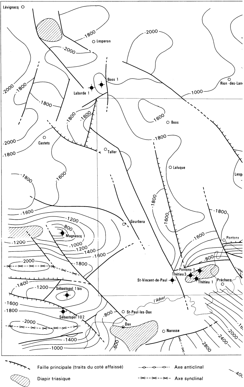
Fig. 5 - Esquisse structur: (dressée à partir des campagnes géoph
