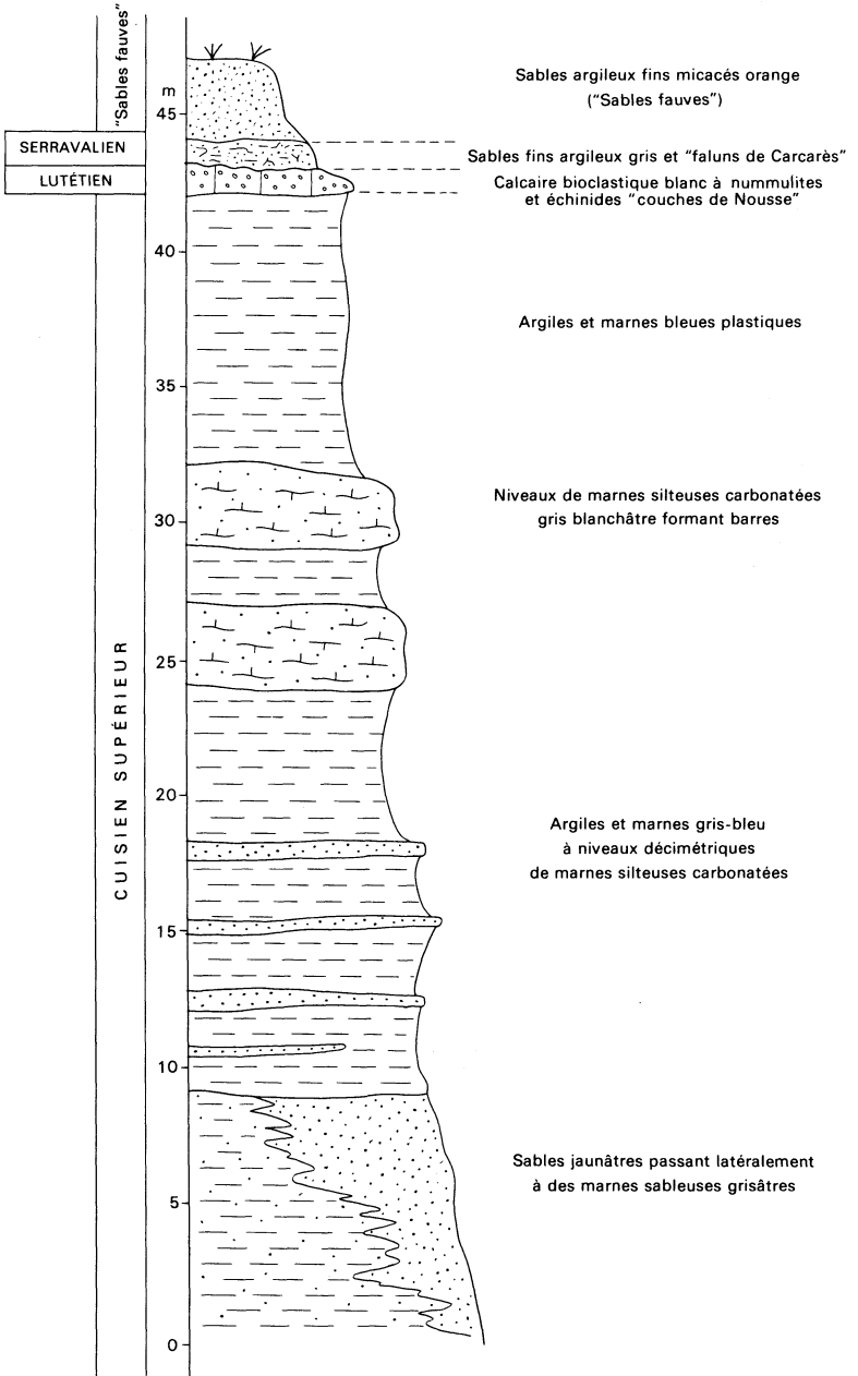
Fig. 1 - Grande carrière de la tuilerie de Saint-Géours-d'Auribat
